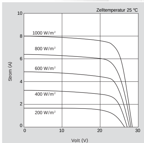
Strom-Spannungs-Kennlinie des Moduls KC167GH-2 bei verschiedener Einstrahlung.
