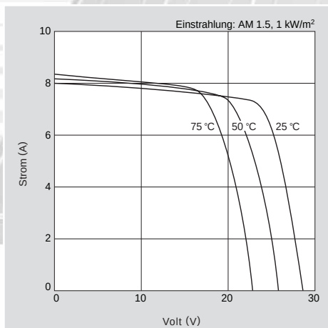
Strom-Spannungs-Kennlinie des Moduls KC167GH-2 bei verschiedenen Zelltemperaturen.
